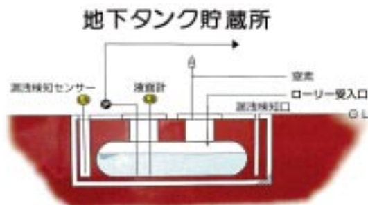
地下タンクの二重化対策（鹿児島川内工場） コンクリートのタンク室内に地下タンクを設置し、漏洩の早期発見及び拡大を防止する構造としている。
