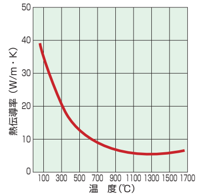
図2 熱伝導率の温度依存性
