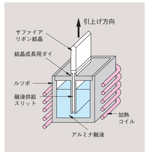
EFG法概念図
