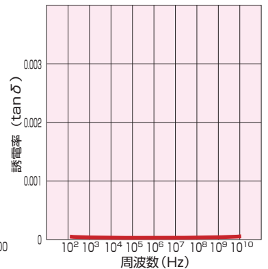
図4 誘電損失の周波数依存性
