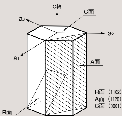
サファイアの単結晶の代表的な面方位
