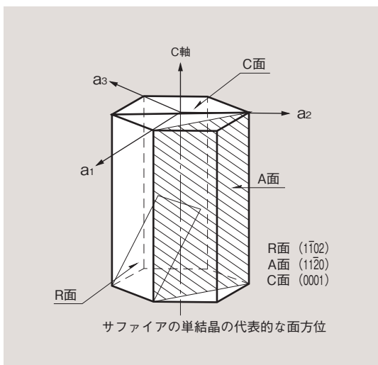
サファイアのユニットセル図
