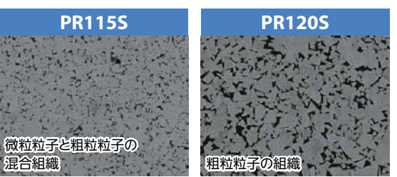
優れた耐熱性を実現 (PR115S) / 優れた耐熱性と安定性を実現 (PR120S)
