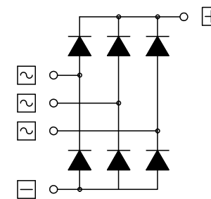
結線図
