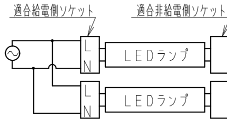
2灯用結線図
