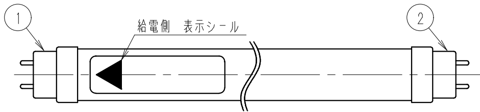
全体図 1/10
