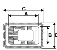
水晶発振器(OSC)用 パッケージ
