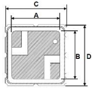
モノリシック水晶フィルタ(MCF)用 パッケージ
