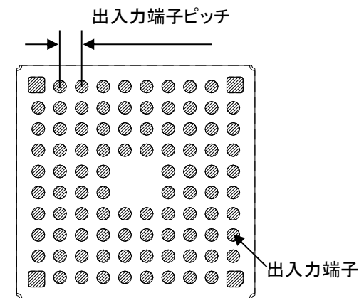
Land Grid Array® Package 「Land Grid Array」は京セラ株式会社の登録商標です。
