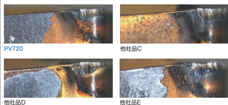
切削時間48分後 逃げ面摩耗状態 (当社比較)
